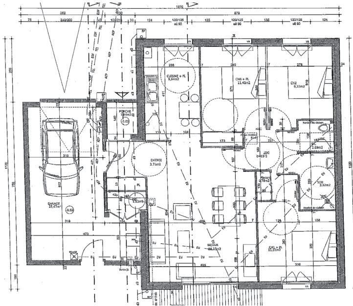
Plan d'un logement
